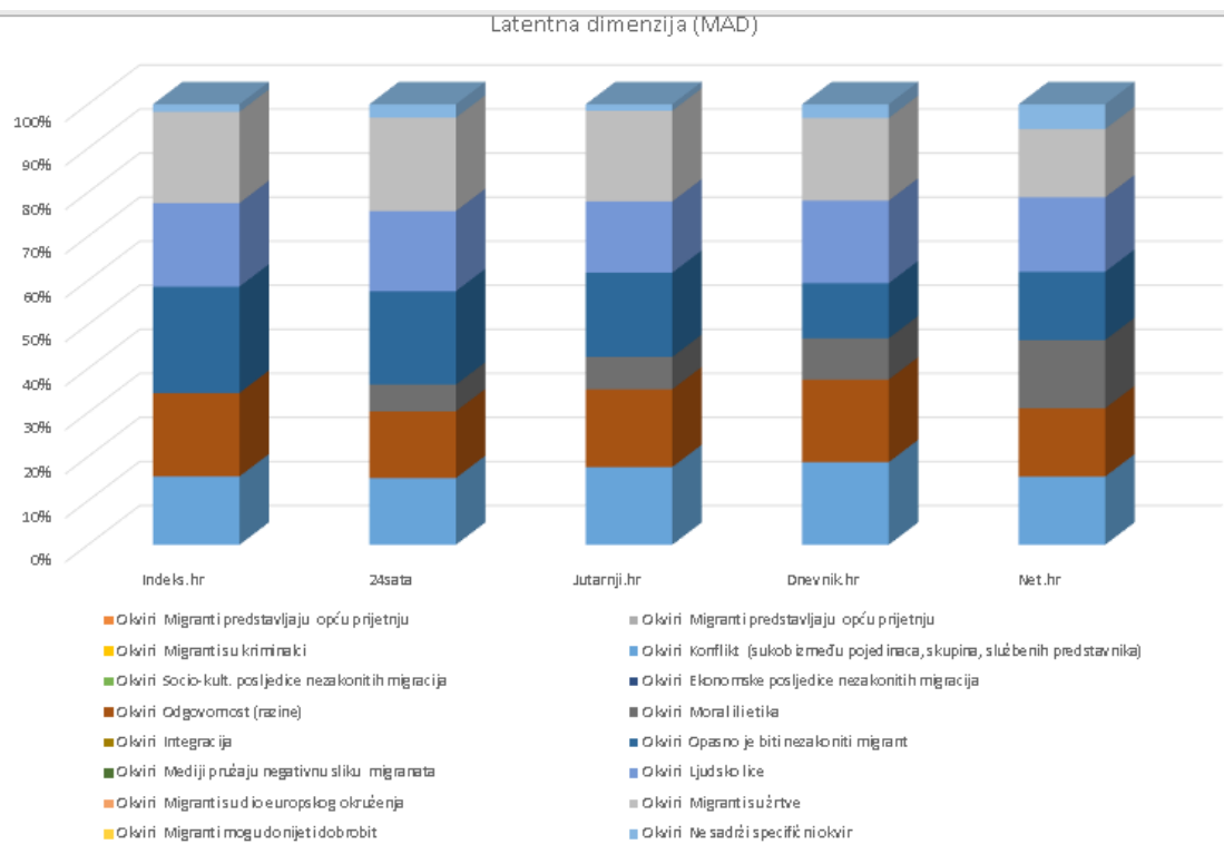
Graf 2. Latentna dimenzija Okviri (MAD)
