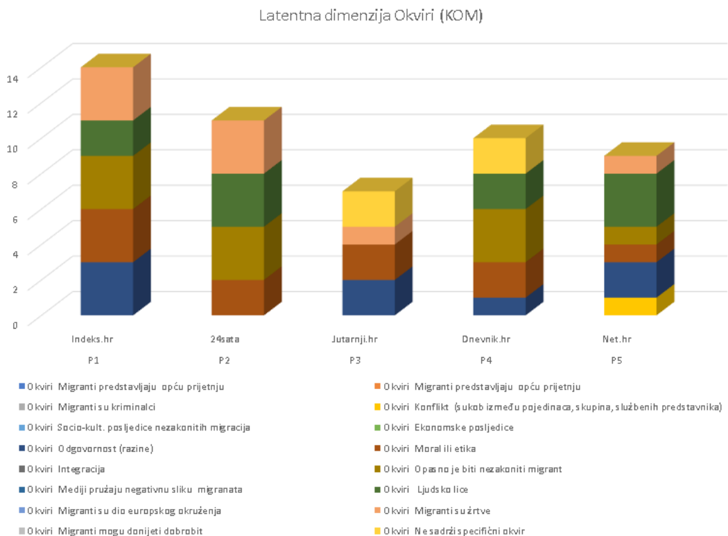
Graf 1. Latentna dimenzija Okviri (KOM)
